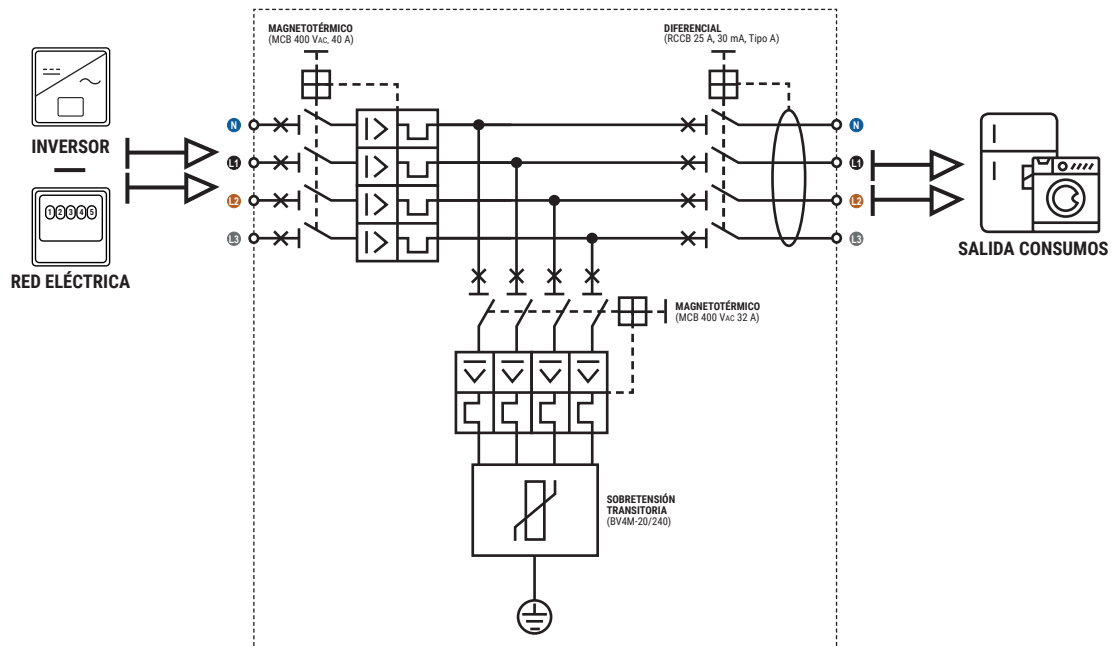
Esquema eléctrico SPAC 4-40
