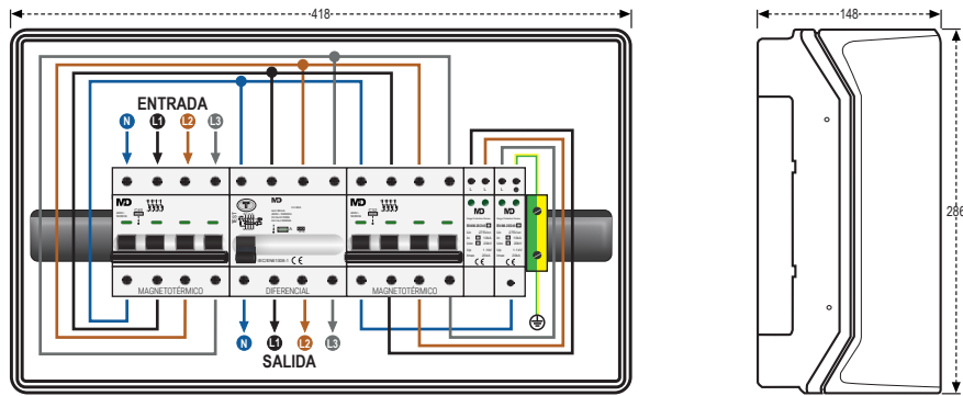
Plano de conexión SPAC 4-40 y Dimensiones
