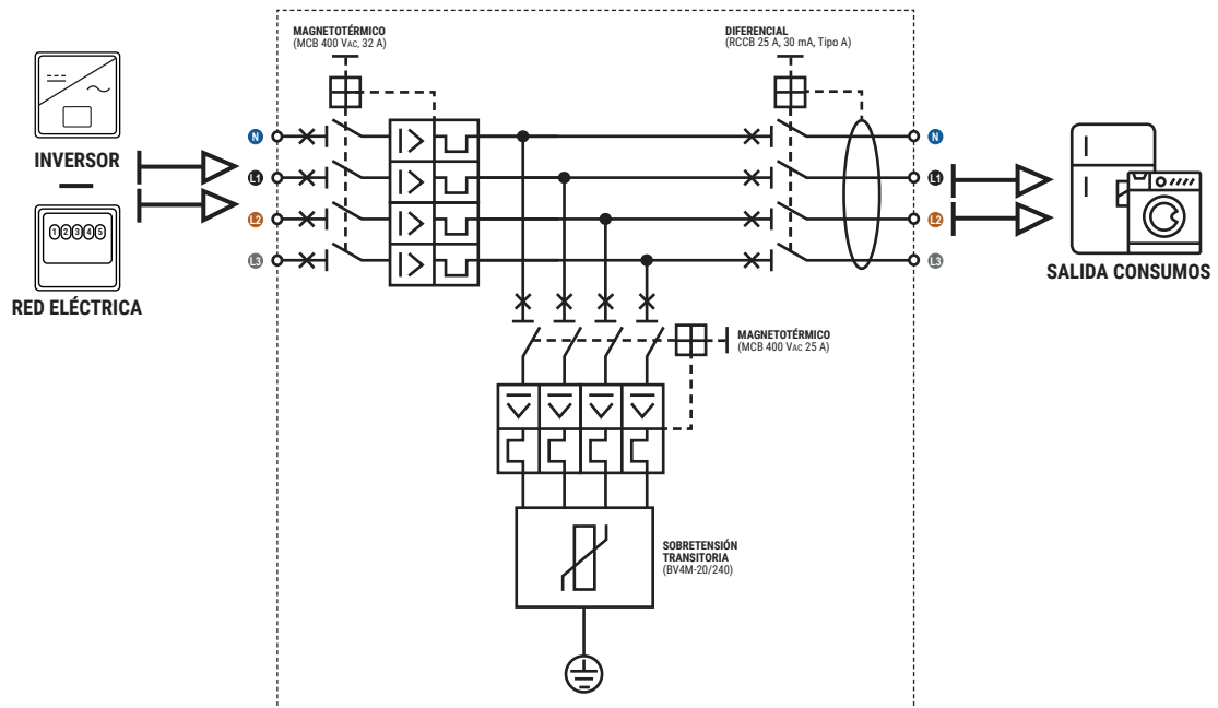
Esquema eléctrico SPAC 4-32
