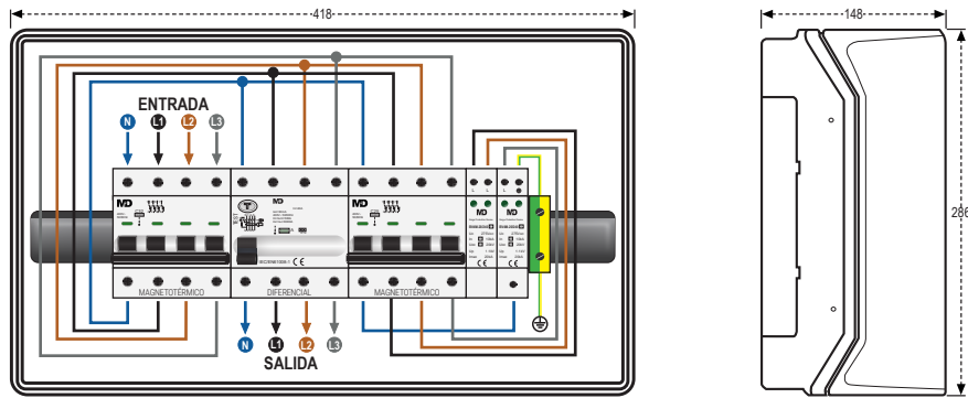
Plano de conexión SPAC 4-32 y Dimensiones
