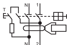
Esquema eléctrico
