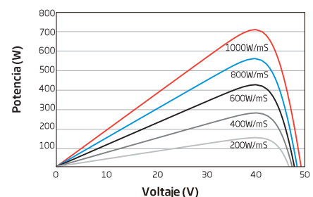
CURVAS P-V CURVES DEL MÓDULO PV (705W)
