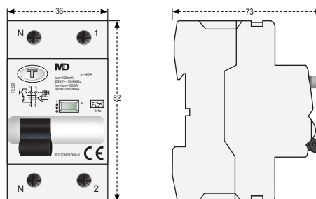
Dimensiones
