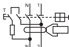
Esquema eléctrico
