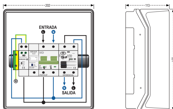
Plano de conexión SPVE 2-32/MLT y Dimensiones
