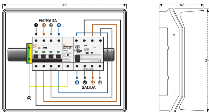
Plano de conexión SPVE 4-32 y Dimensiones
