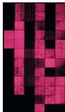
Módulo FV afectado por la PID
