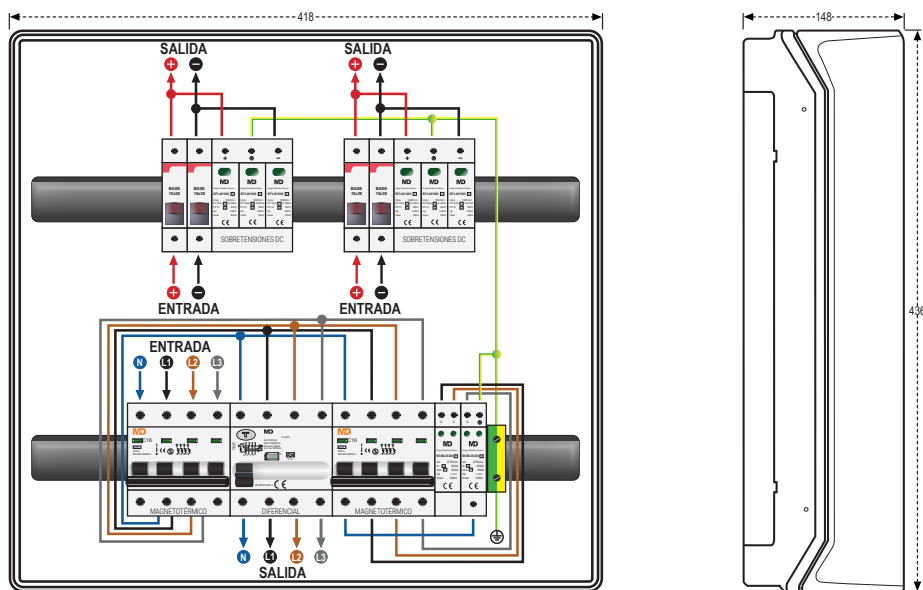
Plano de conexión SPF 2/2-40/1000/20 (223) + AC4-16 y Dimensiones
