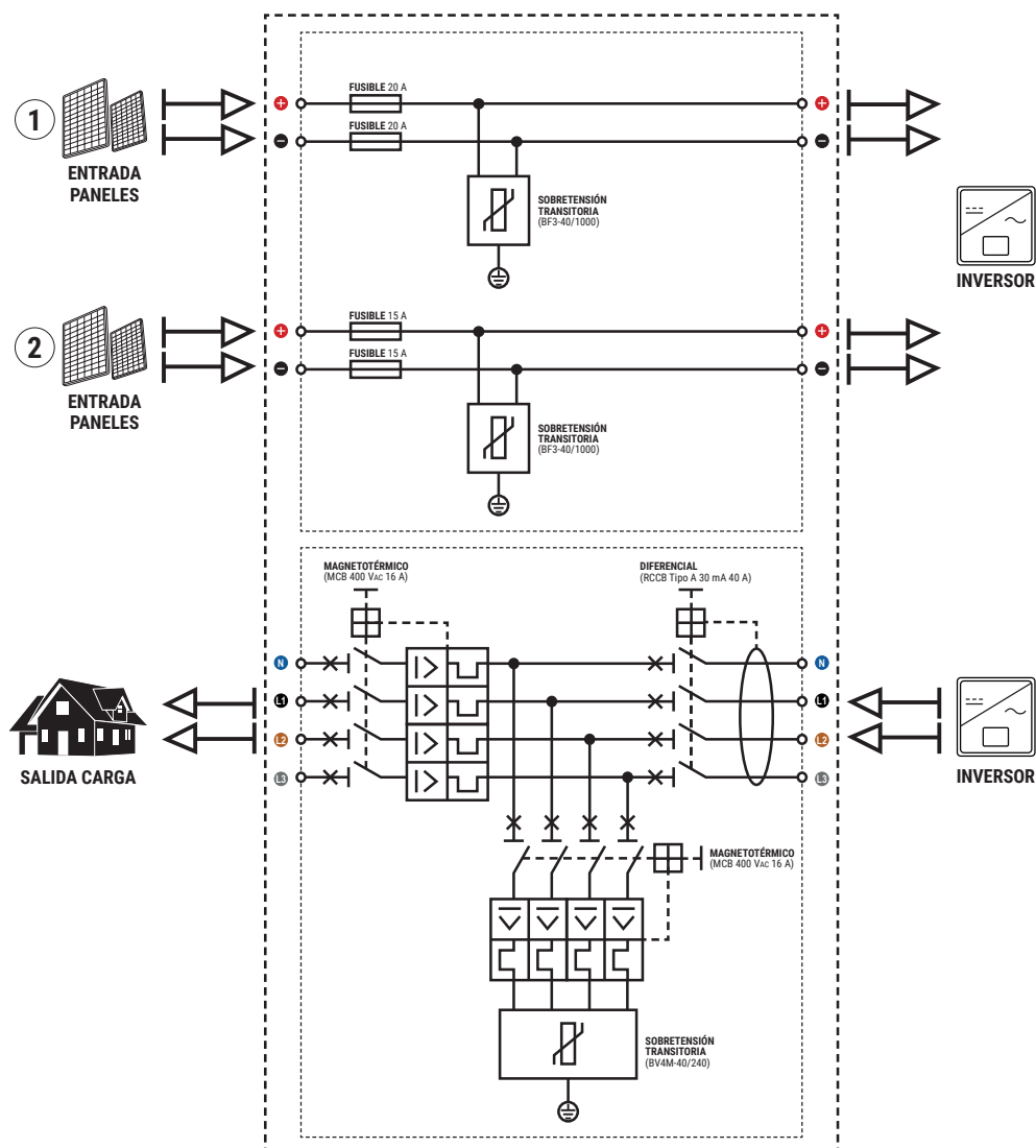
Esquema eléctrico SPF 2/2-40/1000/20 (223) + AC4-16
