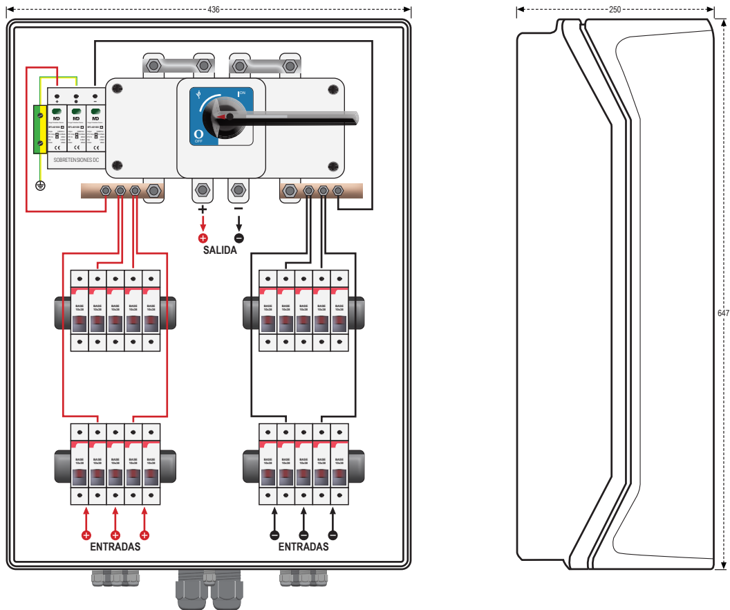
Plano de conexión SPF 10/1-40/1000/15 (122) y Dimensiones
