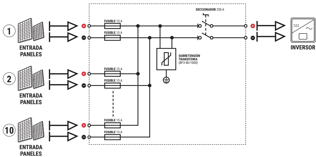
Esquema eléctrico SPF 10/1-40/1000/15 (122)
