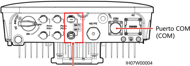
Bornes de la batería (BAT+/BAT-)
