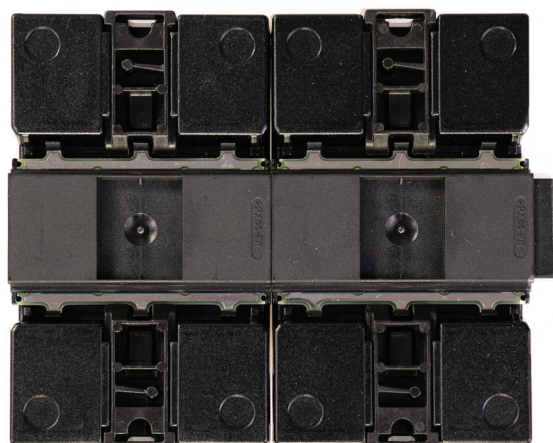
Fig.: Solar-Log™ Base y Solar-Log™ MOD 485 con conectores de bus ensamblados
