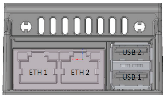
Fig.: Conexiones de la parte inferior del Solar-Log™ Base
