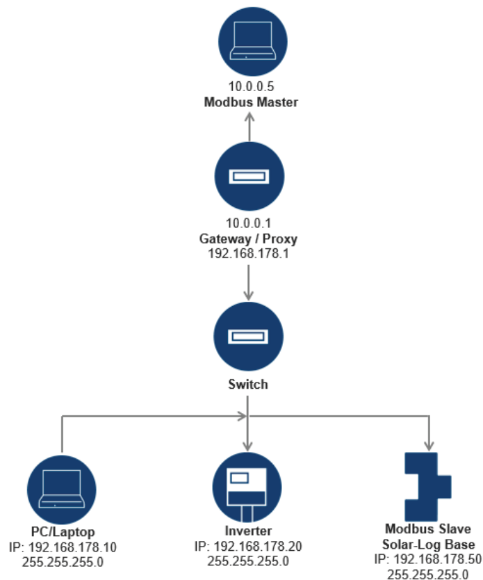
Fig.: Ejemplo de ruta estática
