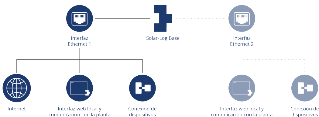
Fig.: Ejemplo con la interfaz de ethernet 1 activada y la interfaz de ethernet 2 desactivada
