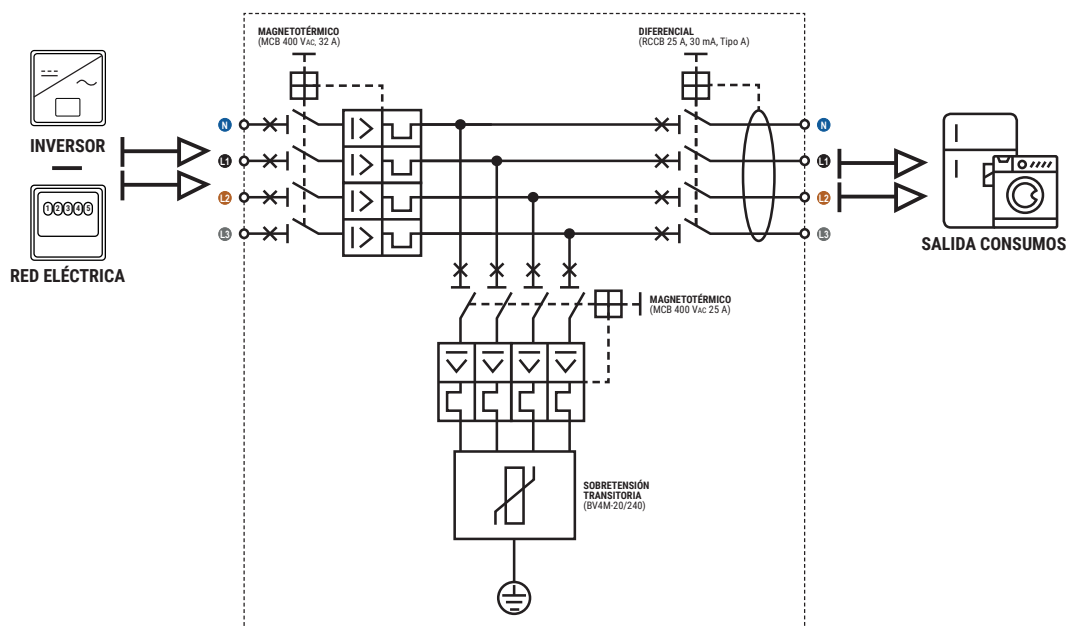
Esquema eléctrico SPAC 4-32
