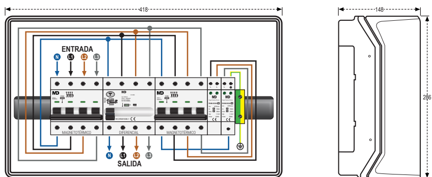
Plano de conexión SPAC 4-32 y Dimensiones
