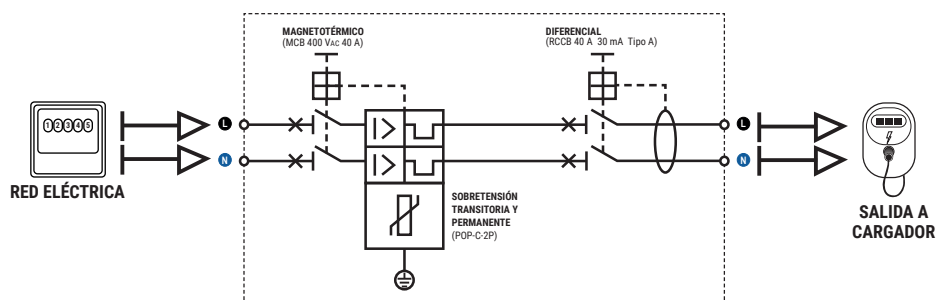
Esquema eléctrico SPVE 2-40
