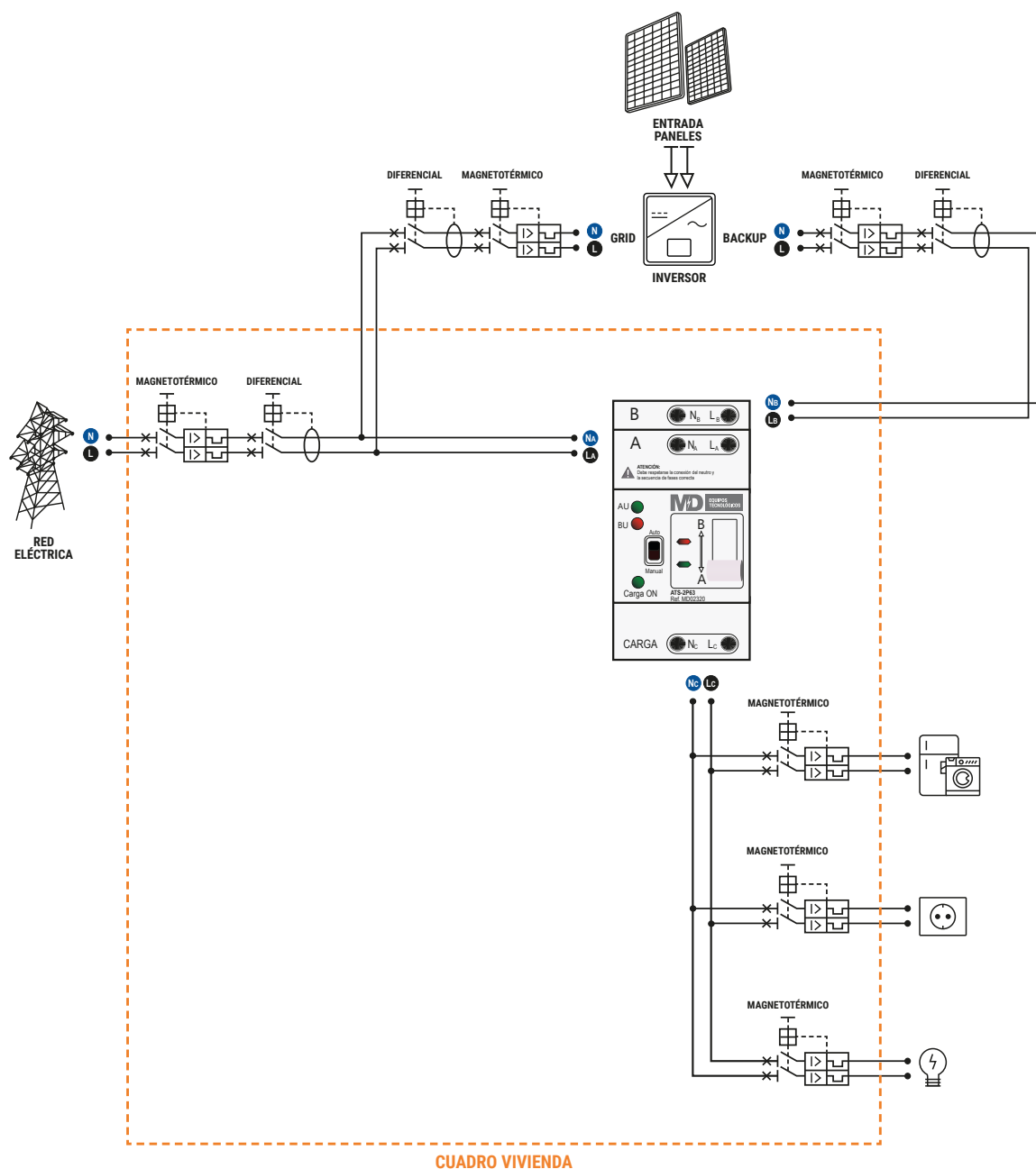
CUADRO VIVIENDA Esquema eléctrico ATS-2P63
