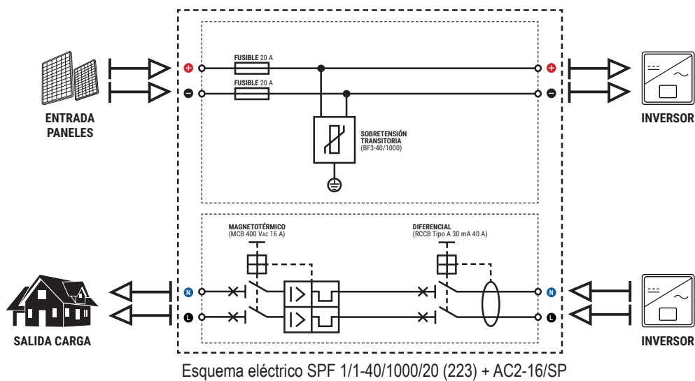
Plano de conexión SPF 1/1-40/1000/20 (223) + AC2-16/SP y Dimensiones
