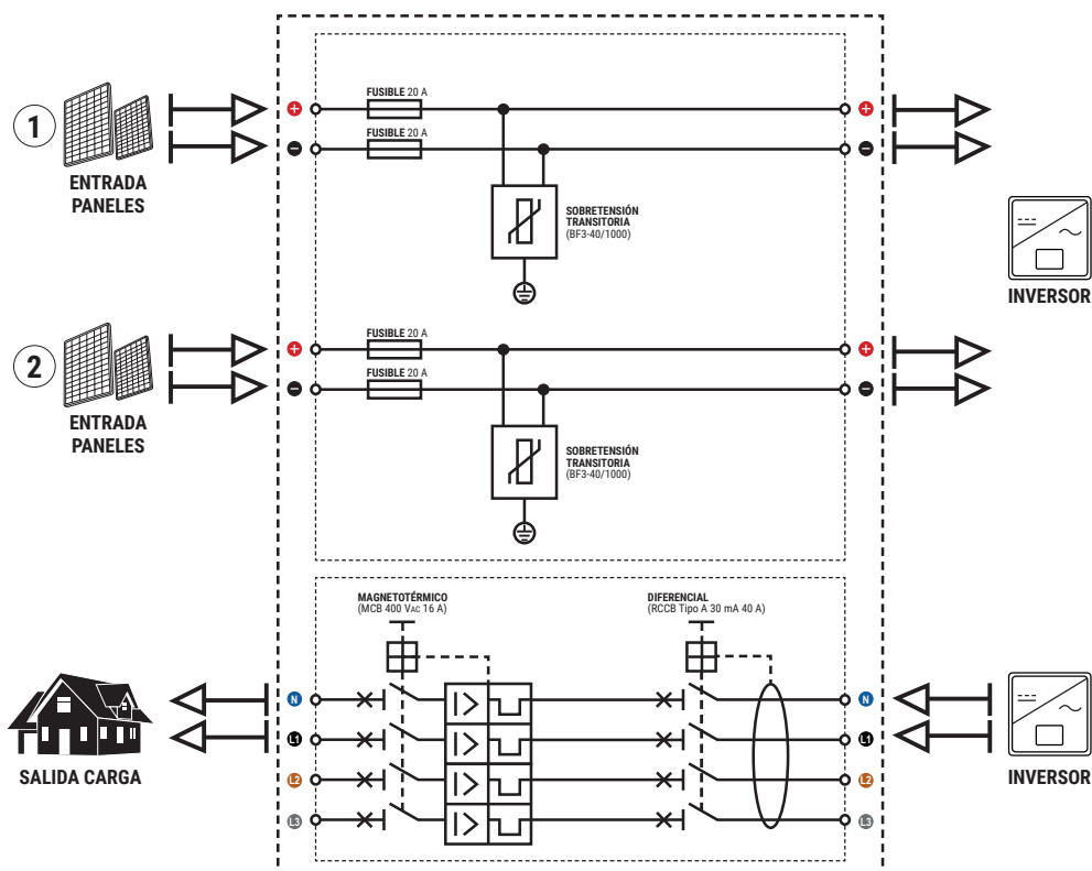
Esquema eléctrico SPF 2/2-40/1000/20 (223) + AC4-16/SP
