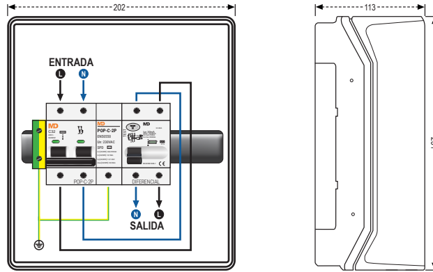
Plano de conexión SPVE 2-32 y Dimensiones
