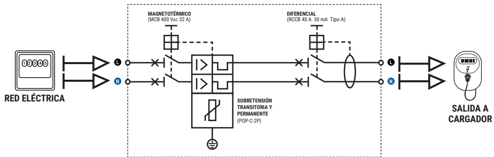
Esquema eléctrico SPVE 2-32
