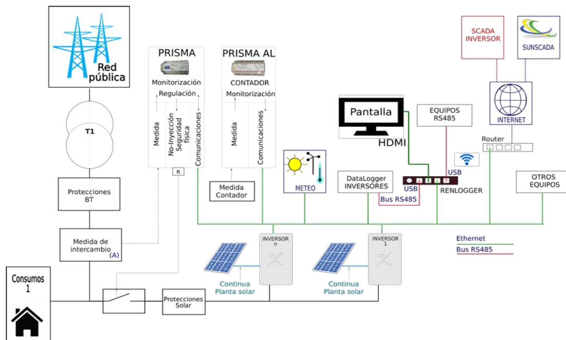
Figura 2 Esquema tipo instalación autoconsumo con RENLOGGER y varias soluciones de integración de equipo
