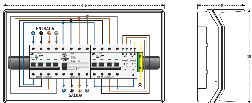
Plano de conexión SPAC 4-40 y Dimensiones
