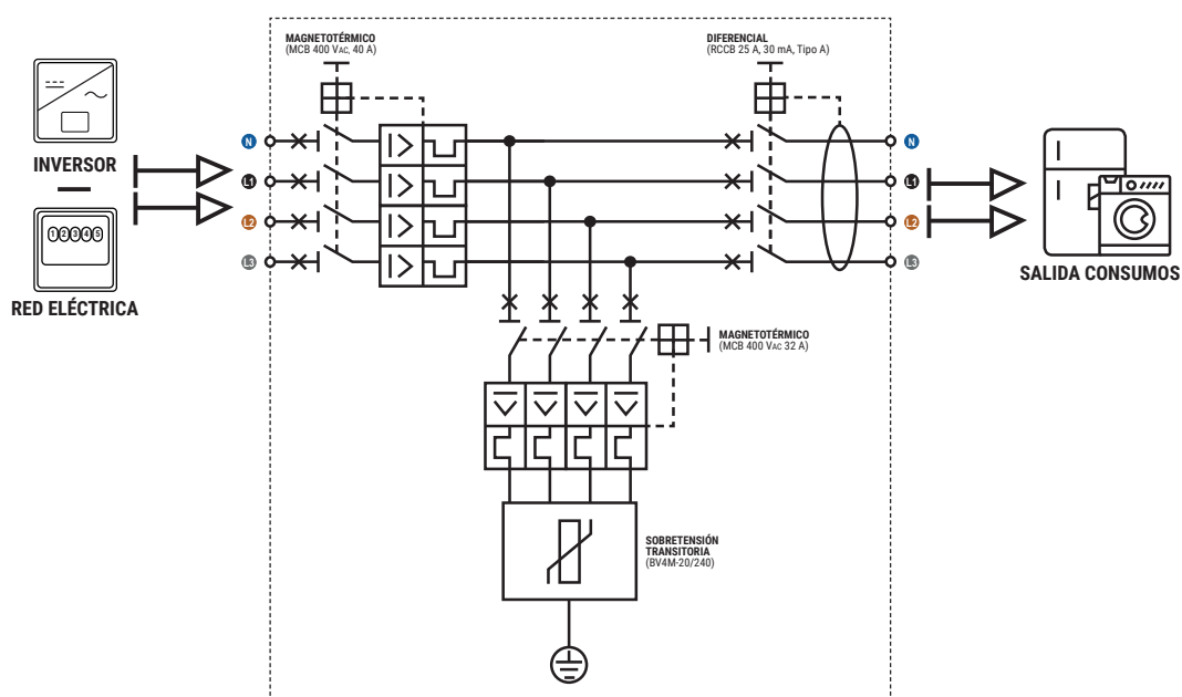
Esquema eléctrico SPAC 4-40
