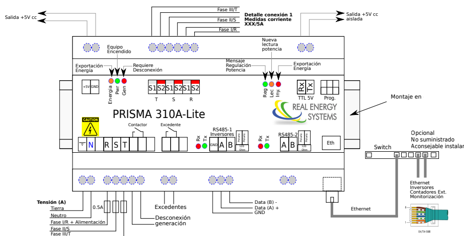
Figura 2 Esquema Unifilar
