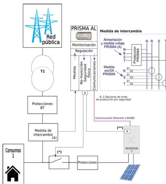
Figura 2 Esquema Unifilar
