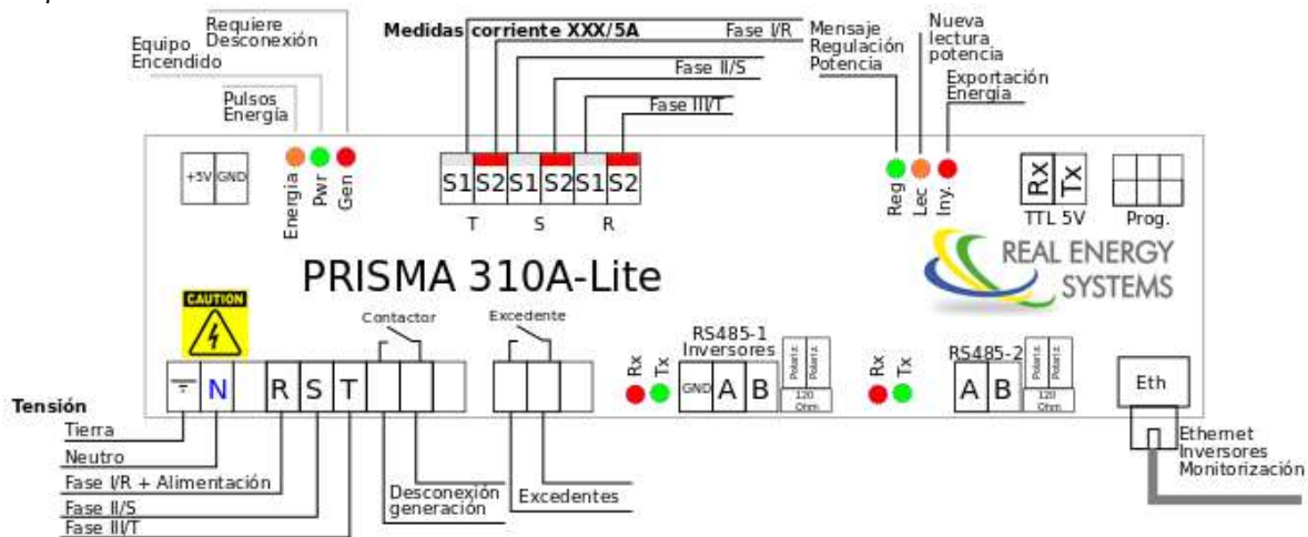
Ilustración 1: Esquema de conexiones y leyenda de indicadores
